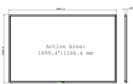
87" 16:10, TABLEAU BLANC INTERACTIF
